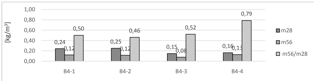
Rysunek 4. Suma złuszczonego betonu B4 (CEM II/B-V, AEA naturalna, w/c = 0,45 po 28 i 56 cyklach zamrażania-rozmrażania w obecności soli odladzających oraz ilość złuszczonego betonu po 56 cyklach w stosunku do ilości po 28 cyklach. Kategoria FT2.
