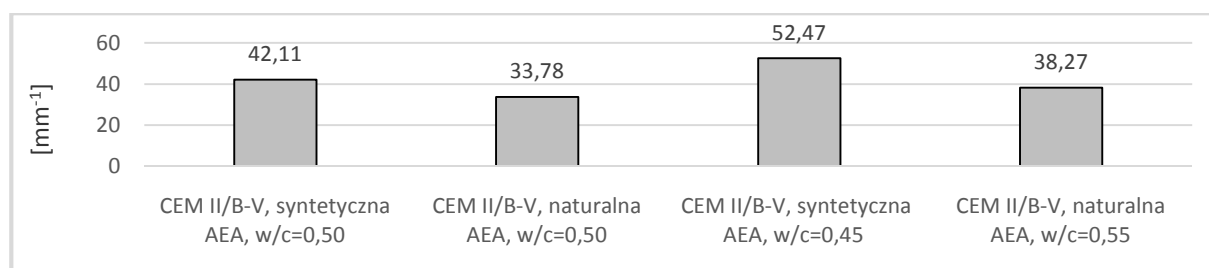
Rysunek 10. Powierzchnia właściwa porów (α) w betonie.
