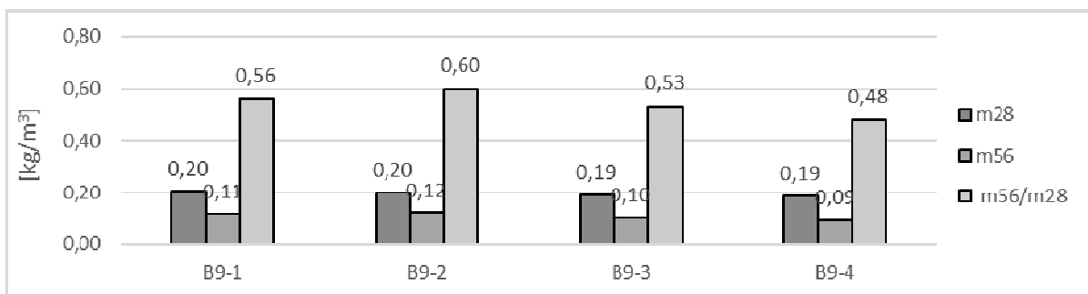
Rysunek 5. Suma złuszczonego betonu B9 (CEM II/B-V, AEA syntetyczna, w/c = 0,55) po 28 i 56 cyklach zamrażania-rozmrażania w obecności soli odladzających oraz ilość złuszczonego betonu po 56 cyklach w stosunku do ilości po 28 cyklach. Kategoria FT2.
